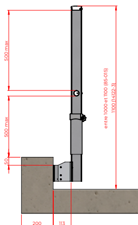
Applicque déporté 110 mm
