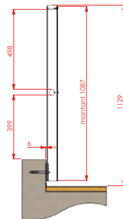
Droit, simple et déporté 80 mm
